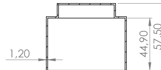
PRZEKRÓJ A-A
