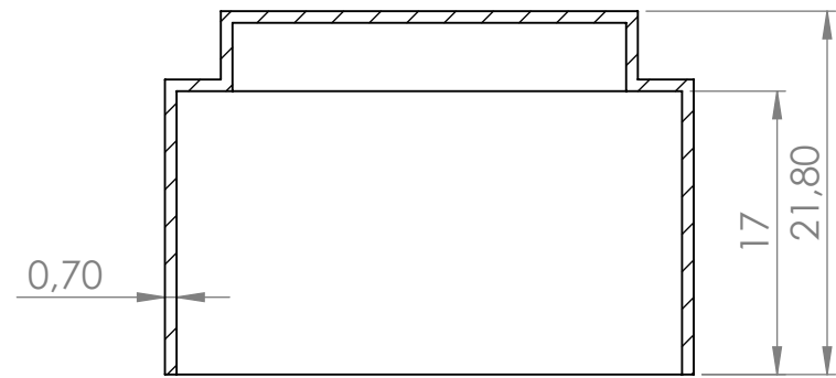
PRZEKRÓJ A-A
